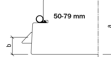
Detalj 5
